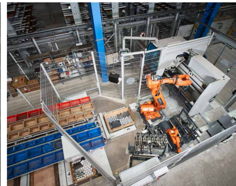
Scie circulaire KASTO intégrée avec KASTOsort.
