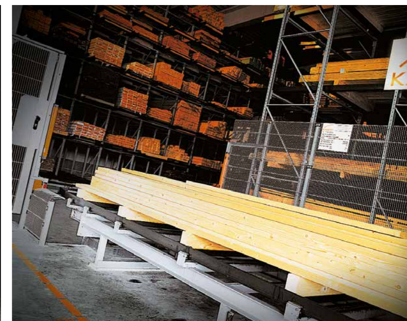
Transstockeur avec dispositif de traction pour le transport sécurisé des cassettes.
