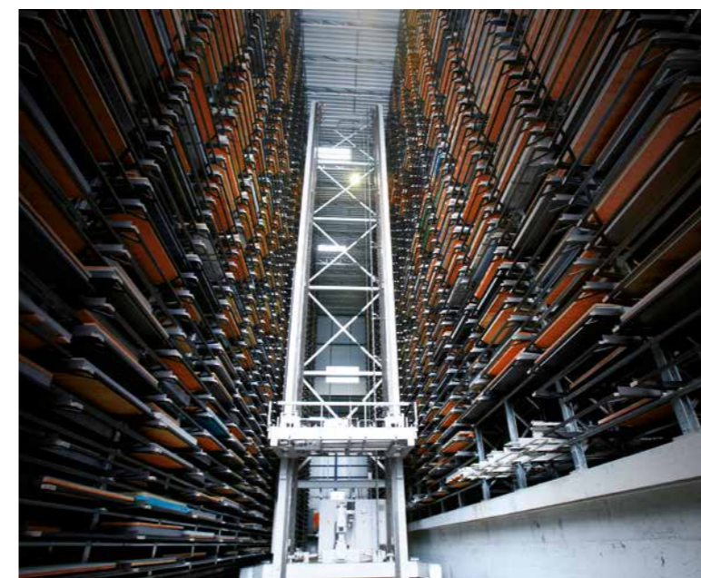
La barrière immatérielle et l'axe laser assurent une transmission précise des données et un positionnement précis du transstockeur
