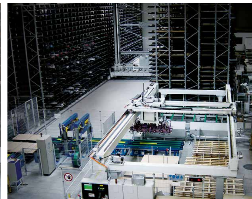
L'appareil de préparation de commandes permet un prélèvement ergonomique et rapide de la matière.
